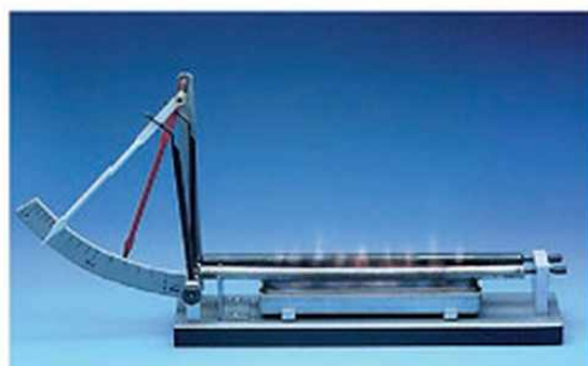
128.2. Különböző fémek hőtágulása azonos feltételek mellett is különböző.
