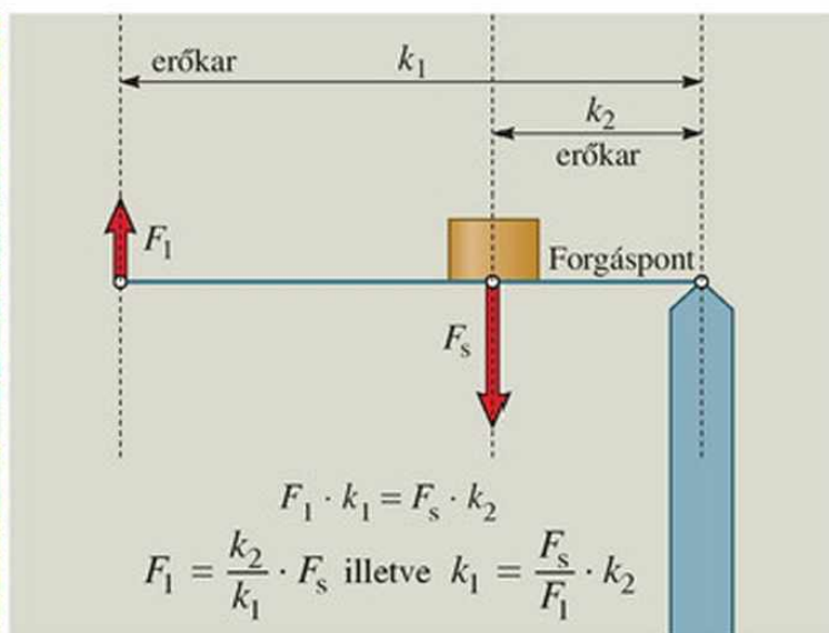
103.5. Egyoldalú emelőknél az erők támadáspontja a forgástengely ugyanazon oldalán van.
