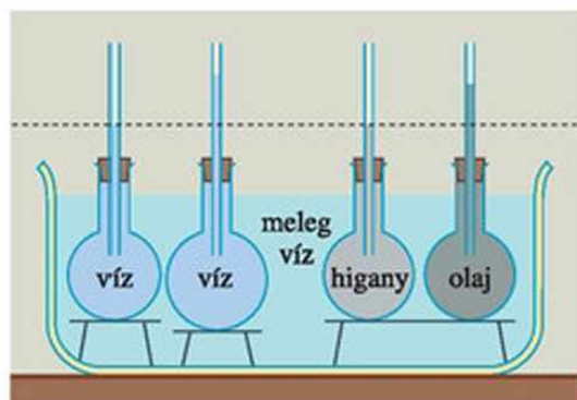
126.1. A folyadékok hőtágulásának mértéke az anyagi minőségtől és a kezdeti térfogattól függ, ha a hőmérséklet-változás azonos.
