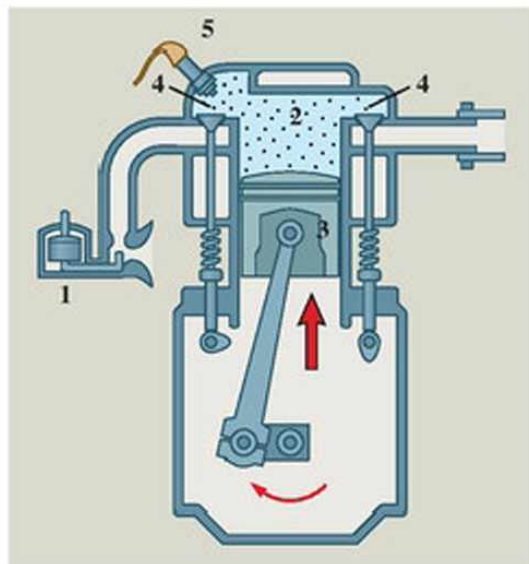
142.1. Benzinmotor metszeti rajza. Porlasztó (1); munkahenger (2); dugattyú (3); szelepek (4); gyújtógyertya (5).
