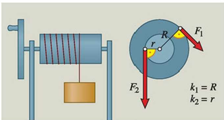
104.3. Az egyensúlyban levő hengerkeréknél: F_1 \cdot R = F_2 \cdot r . Ebből kiszámítható az egyensúlyt létrehozó erő:
