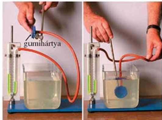
78.3. A legegyszerűbb manométer.
