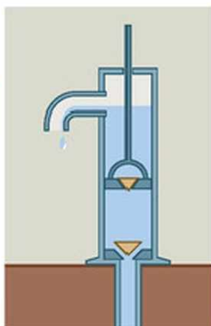
szívókút
