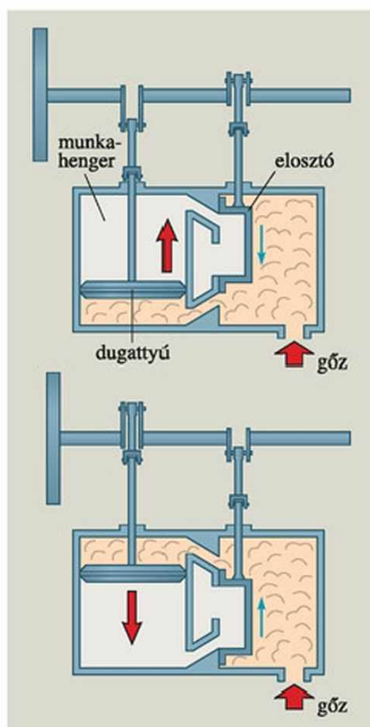
141.1. A Watt-féle gőzgép modelljének metszeti rajza
