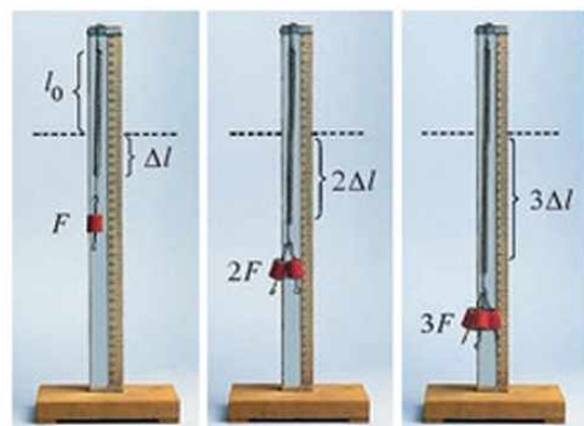
58.1. Minél nagyobb a feszítőerő, annál nagyobb a rugó megnyúlása.
