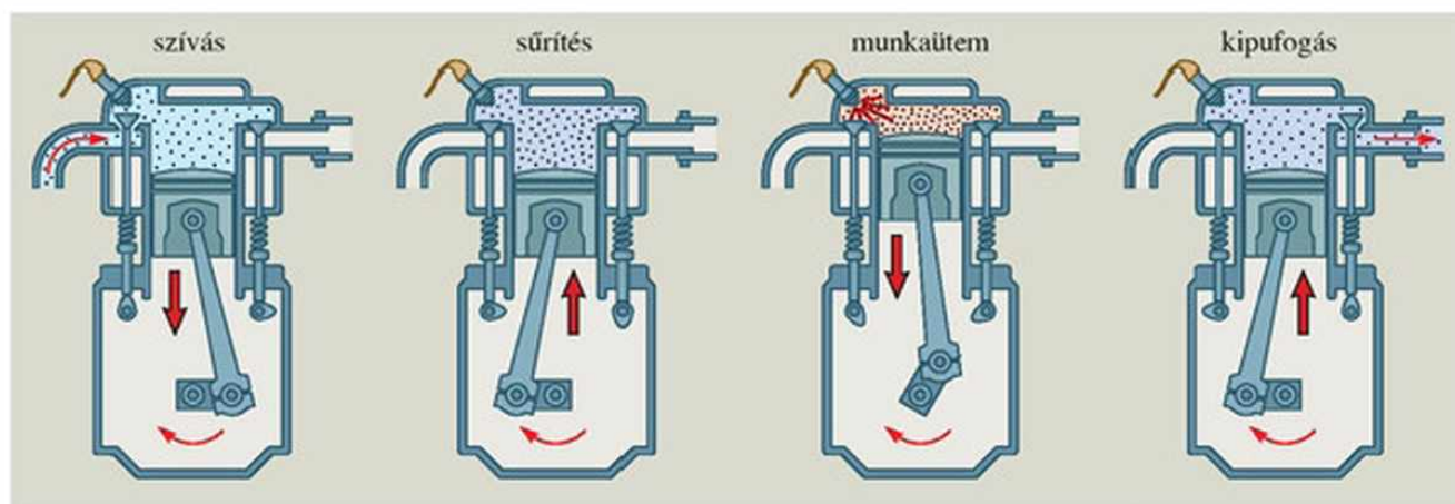
142.3. A négyütemű benzinmotor működésének jellegzetes szakaszai.
