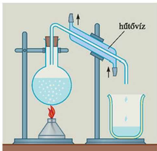
134.3. Desztilláláskor a vízgőz lecsapódik.
