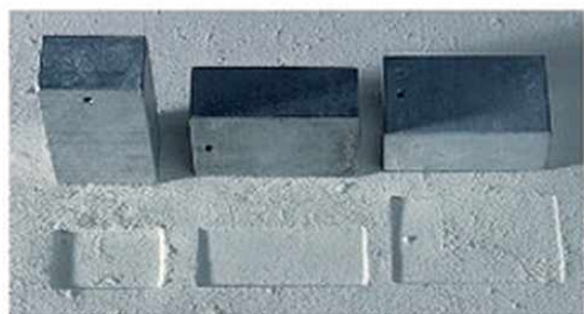
74.2. Egyenlő nyomóerő, de különböző nyomott felület esetén más a benyomódás mértéke.
