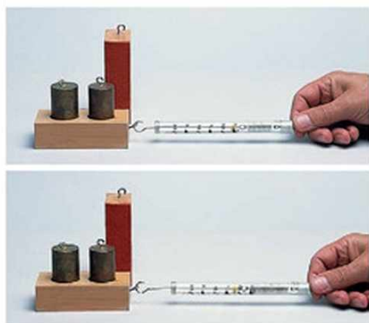
64.1. Bár a hasábot húzzuk, a tapadás miatt mégsem mozdul el.
