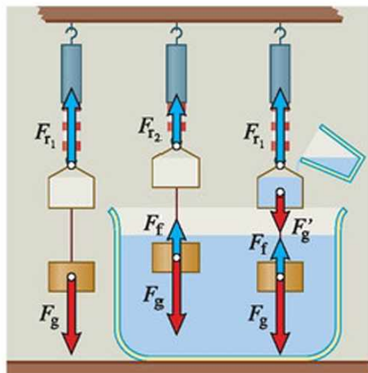
87.2. A víz által kifejtett felhajtóerő egyenlő a hengerbe töltött víz súlyával.
