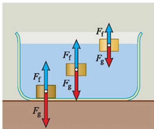
89.2. Ha a test nagyobb sűrűségű, mint a folyadék, akkor elmerül benne. Ha a test és a folyadék sűrűsége egyenlő, a test lebeg. Ha a test sűrűsége kisebb, mint a folyadéké, a test csak részben merül a folyadékba, vagyis úszik.
