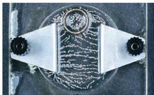
22.2. Az elektromos mező a fémgyűrű hatására megváltozott.
