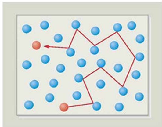
10.3. Miért zezugos a gárrészecskék mozgása?
