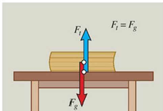
61.1. A nyugalomban lévő könyvre két erő hat: a gravitációs erő és a tartóerő, melyek kiegyenlítik egymást.
