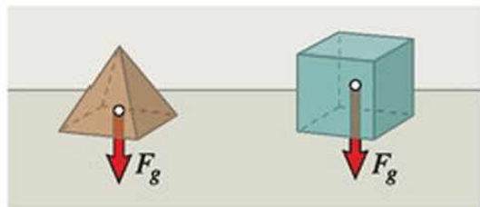
54.3. A gravitációs erő támadáspontját a test középpontjába szoktuk rajzolni.
