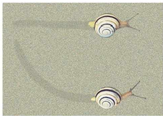
30.2. A mozgás pályája lehet egyenes vagy görbe vonalú.
