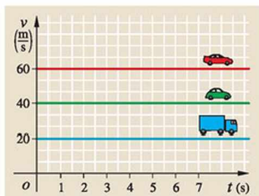
32.1. Az egyenletes mozgást végző test sebessége állandó.
