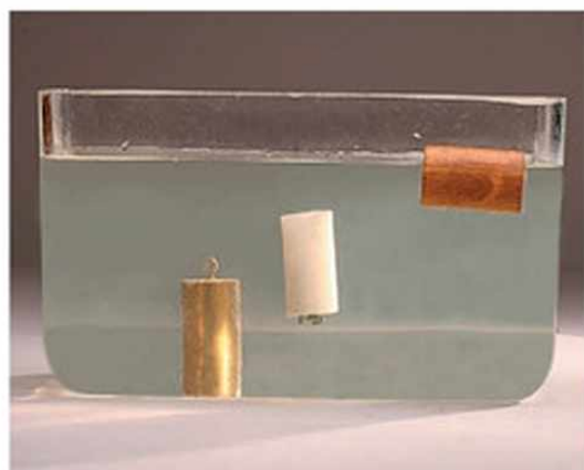
89.1. A fadarab fennmarad a vízben, a réz elsüllyed, a gyertya pedig lebeg benne.
