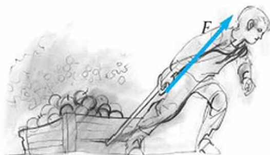
51.3. Mire következtethetünk az erőt ábrázoló nyíl hosszából és irányából?
