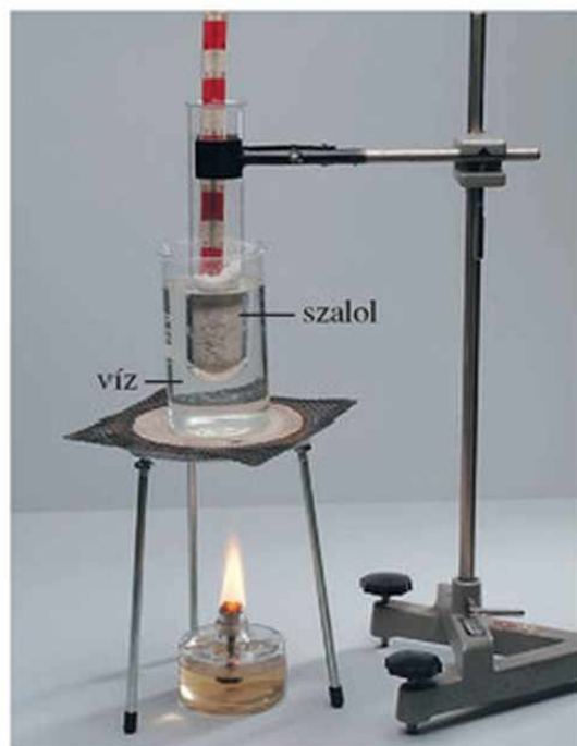
130.1. Az anyag halmazállapota nem állandó.
