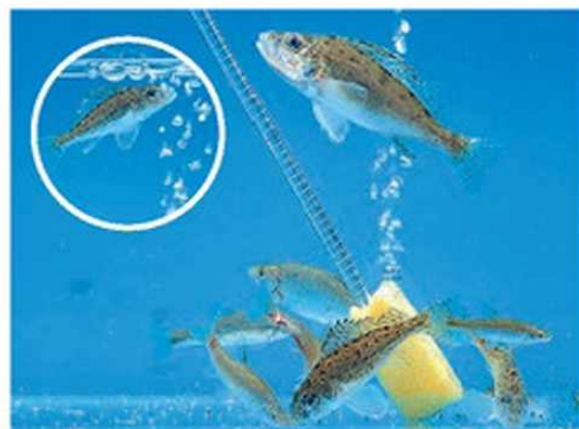
139.2. A vízben oldott oxigén nélkül a halak elpusztulnak.
