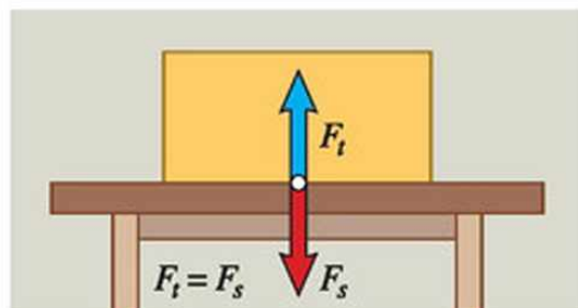
59.4. Az erő és az ellenelő két különböző testre hat. Hasonlítsd össze a nagyságukat és az irányukat!
