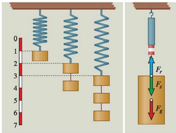
58.3. Mely erőkre lehet következtetni a rugóerő nagyságából?
