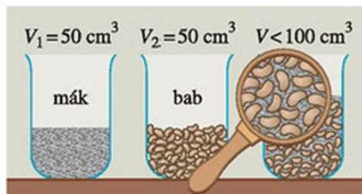
11.2. A folyadékok keveredésének modellezése.
