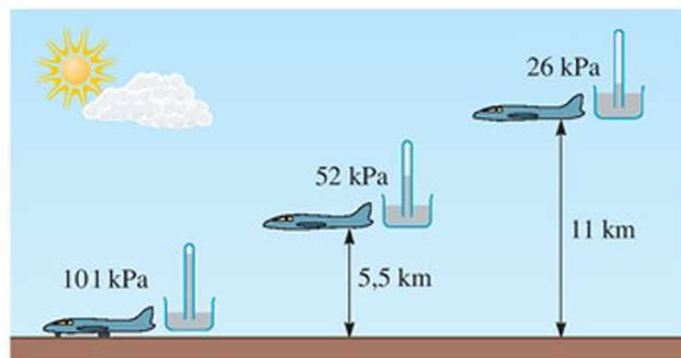
81.4. Miért kisebb a légnomás a magasban, mint a Föld felszínén?
