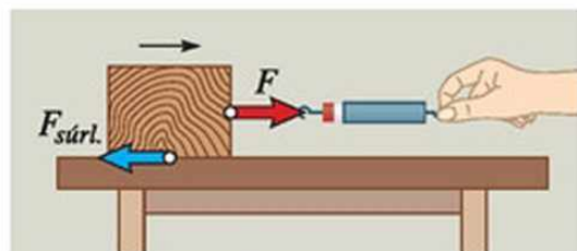
63.3. Egyenletes mozgásnál a súrlódási erő egyenlő nagyságú és ellentétes irányú a húzóerővel.
