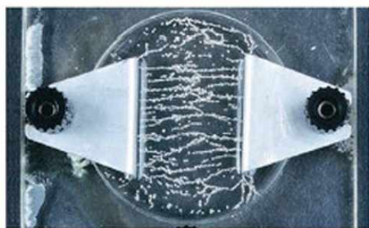
22.1. Minek a hatására rendeződött el vonalak mentén a búzadara?
