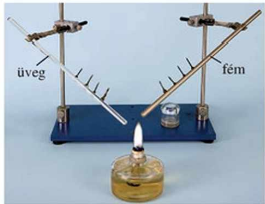
124.3. A szöveget tartó viasz melegítéskor megolvad. A fémrúdról a szögek sorban leesnek, és jelzik az állapotváltozás terjedését.
