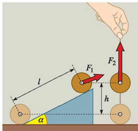
105.3. A két munka egyenlő: F_1 \cdot l = F_2 \cdot h .
