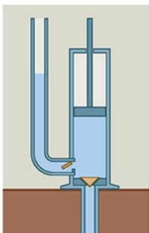
nyomókút
