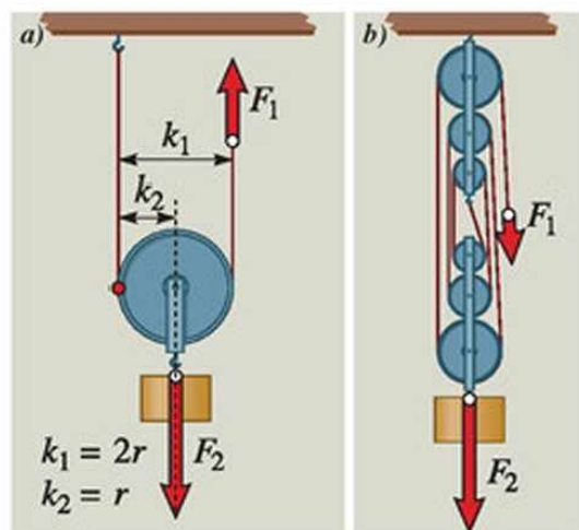
104.4. A mozgócsiga (a) egyoldalú emelő, amelynek: k_1 = 2r ; k_2 = r . A közönséges csigasor (b) álló- és mozgócsigákból áll.
