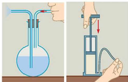
82.3. A gáz nyomása növelhető a részecskeszám növelésével, illetve a térfogat csökkentésével.
