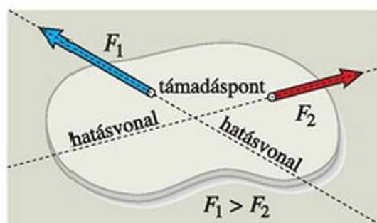
52.1. Ahányszor nagyobb az egyik erő a másikonál, annyszor hosszabb az azt jellemző nyíl a másikat jellemző nyílnál.
