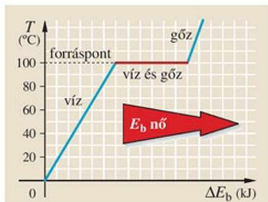
133.3. Forrás közben a folyadék hőmérséklete nem változik.
