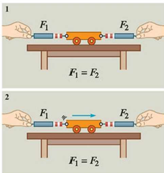
61.2. A kiskocsi egyensúlyban van akkor is, ha áll (1), és akkor is, ha állandó sebességgel mozog (2).
