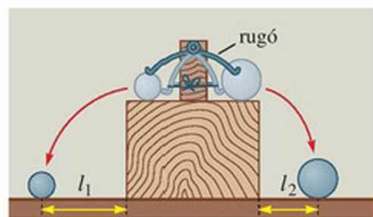
45.2. Akkor azonos a sebességváltozás feltétele, ha mindkét testet egyenlő nagyságú erőhatás egyenlő ideig ér.
