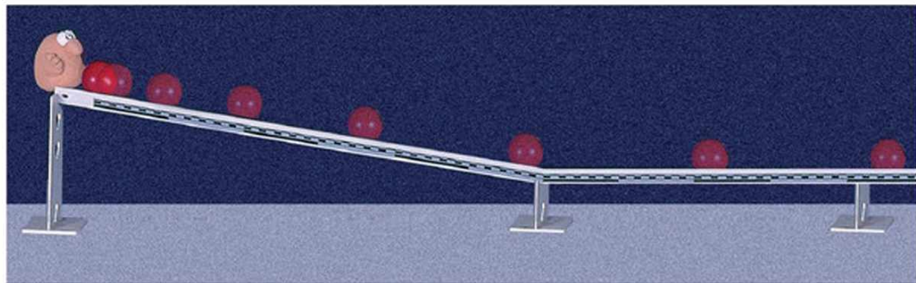
37.1. A lejtőn guruló golyó sebessége változik.
