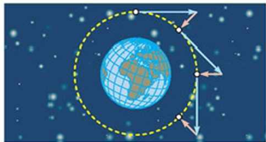
56.2. Az űrhajó „körbeesi” a Földet.
