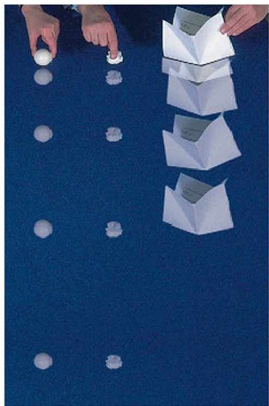
38.3. Mit mutat meg ez a sorozatfelvétel a különféle testek eséséről?
