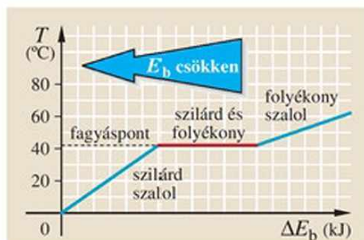
131.3. Fagyás közben az anyag hőt ad le, ilyenkor a hőmérséklete nem változik.
