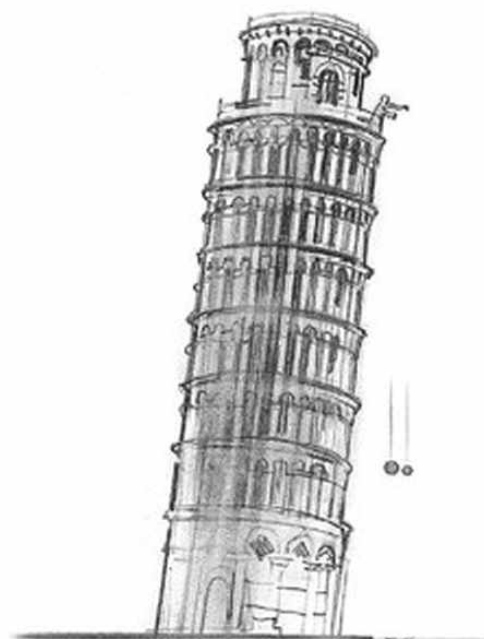
39.2. A szabadesést először Galilei vizsgálta (1600 körül). A legenda szerint a pisai ferde toronyból ejtett le különböző testeket.
