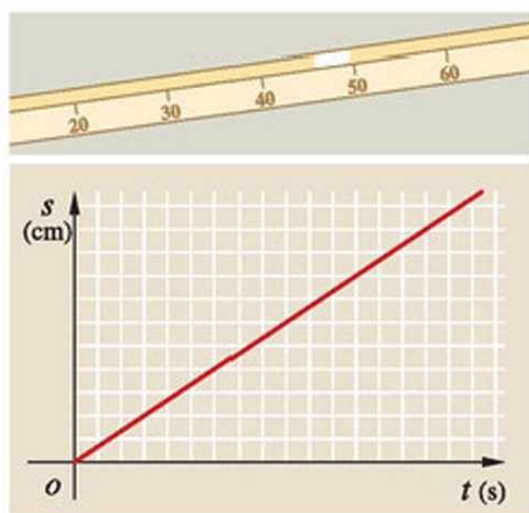
31.1. Ha s \sim t , a mozgás egyenletes.
