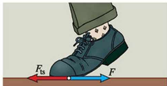
64.2. Lépés közben a láb a súrlódás miatt hátranyomja a földet, a föld előre a lábat (hatás–ellenhatás), ezért tudunk járni.
