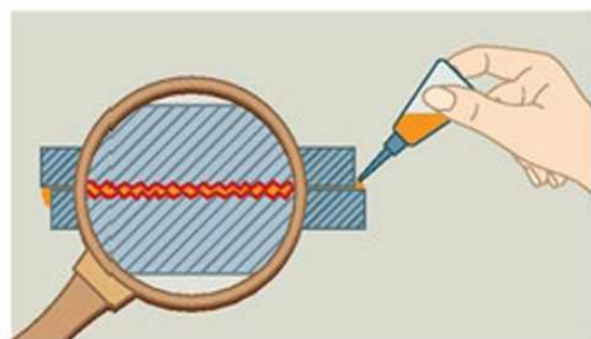
64.3. A kenőanyagok részecskéi könnyen elmozdulnak egymáson.
