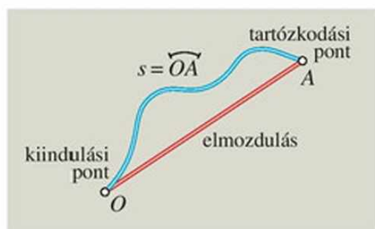
30.4. Miben különbözik egymástól az út és az elmozdulás?
