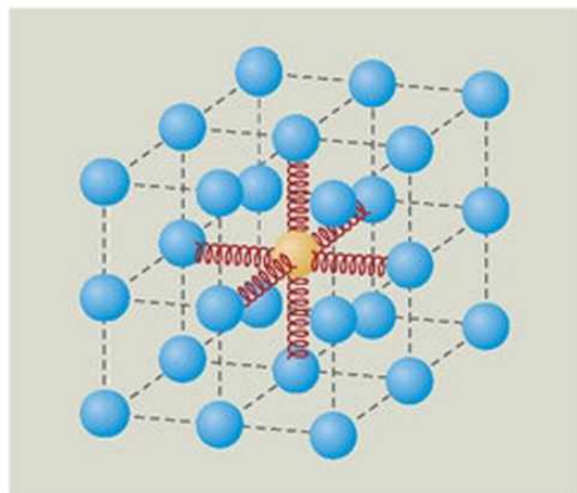
12.1. A szilárd anyag részecskéinek rendszeren rezgését például rugókkal kikötött golyók mozgásával szemléltethetjük, modellezhetjük.
