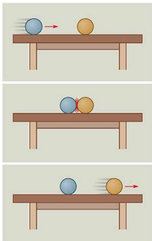
18.1. Milyen hatás következtében változhat meg egy test mozgásállapota?
