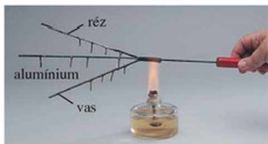
125.1. A rézben gyorsabban terjed az állapotváltozás, mint a vasban.
