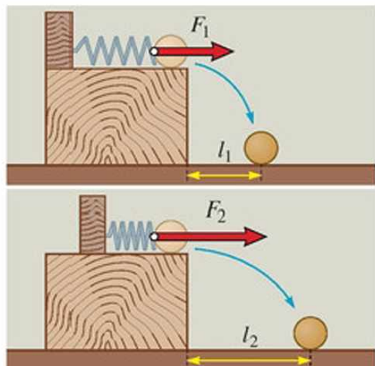
56.4. A jobban megfeszített rugó nagyobb sebességváltozást hoz létre ugyanazon a testen.
