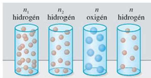
47.1. Egyenlő térfogatú tartályban különböző számú és tömegű gázrészecskék is lehetnek. Ezért a gázok sűrűsége is különböző lehet.
