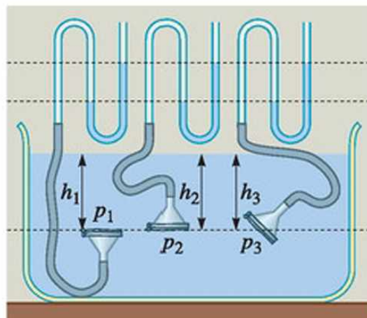
79.1. Ha h_1 = h_2 = h_3 , akkor p_1 = p_2 = p_3 .
