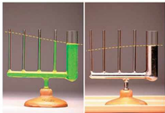
86.1. Minél vékonyabb az üveg hajszálcso, annál magasabban van benne a víz felszíne, és annál alacsonyabban a higanyé.
