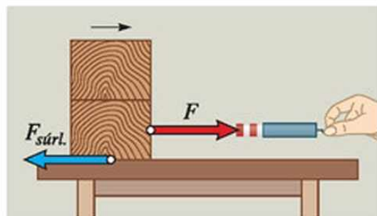
63.4. A súrlódási erő a felületeket összenyomó erő nagyságától is függ.
