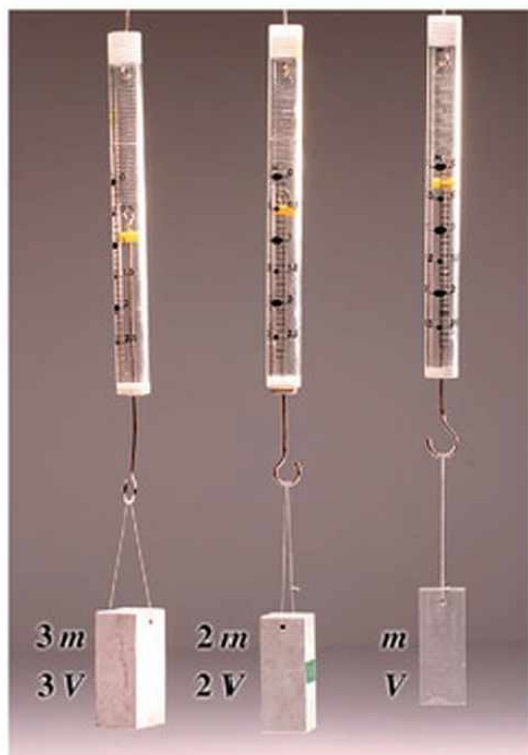
47.2. A megegyező anyagú, homogén testek tömege és térfogata egyenesen arányos.
