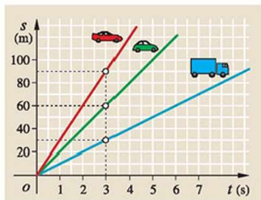
31.2. Mikor meredekebb az egyenletesen mozgó test út-idő grafikonja?
