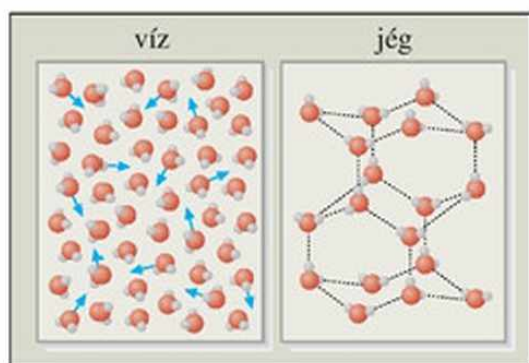
132.1. A jégkristályban a vízmolekulák távolabb vannak egymástól, mint folyékony halmazállapotban.
