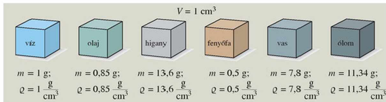
48.1. Különböző anyagok sűrűsége különböző.
