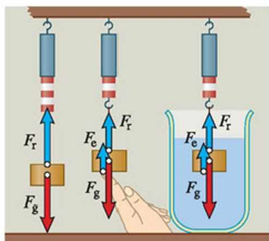
87.1. A gravitációs erőt a rugalmas erő és az emelőerő együttesen egyenlíti ki.
