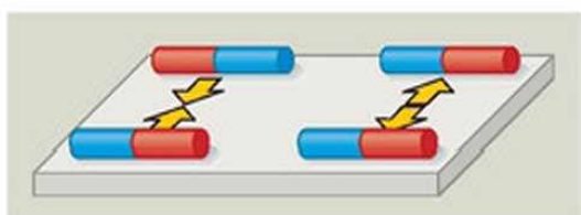
21.3. Miben nyilvánulhat meg a mágneses kölcsönhatás?
