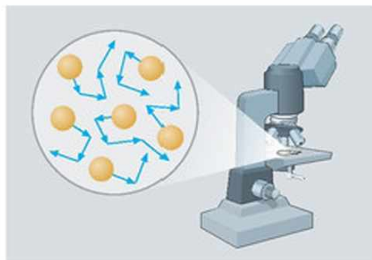
11.4. A Brown-féle mozgás mikroszkóppal jól megfigyelhető.
