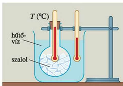
131.2. Fagyás közben a szalol belső energiája csökken, a hűtővizé nő.
