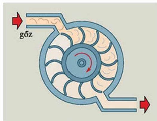
141.2. Az áramló gőz közvetlenül hozza forgásba a turbina kerekét.
